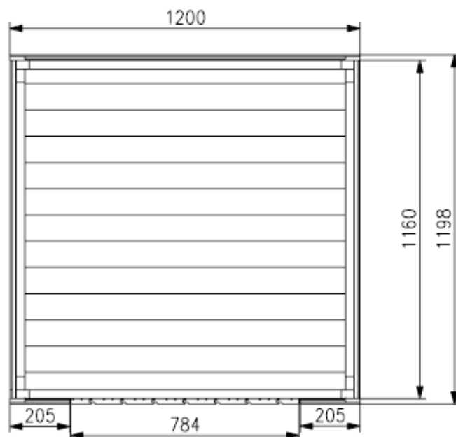
Plan au sol
